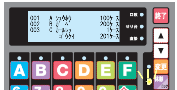
休憩中画面
